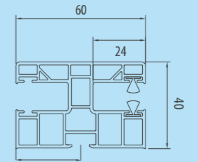
PVC PPD 60/12 Standardführung des Systems Opoterm. Verwendete Schrauben – RD2.
