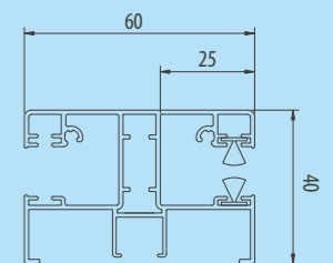
ALU PPDA 60/12 Alu-Äquivalent der Standardführung des Systems Opoterm. Verwendete Schrauben – RD2.
