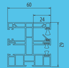
PVC PPDM 60/12 Führung für Rollläden Opoterm mit integriertem Moskitonetz. Verwendete Schrauben – RD2.
